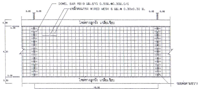
รูปแปลงแสดงการเสริมเหล็กและรอยต่อ
