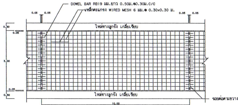
รูปแบบลงการเสริมเหล็กและรอยต่อ
