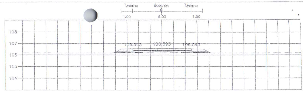
STA. 3+250.000 NGL = 106.185
