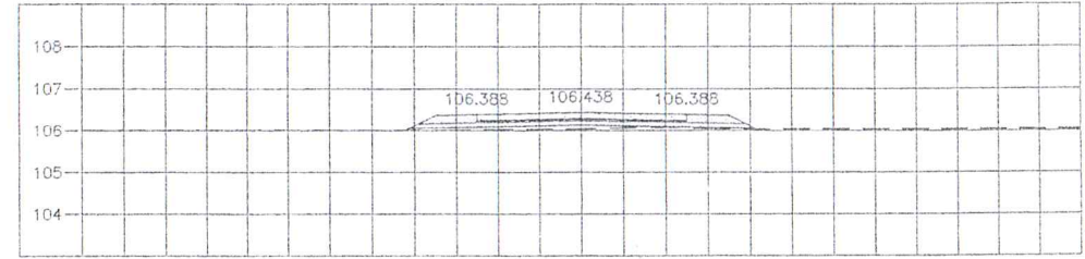
STA. 3+225.000 NGL = 106.045
