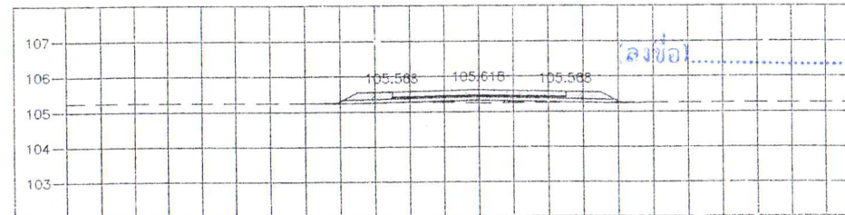
STA. 3+050.000 NGL = 105.245
