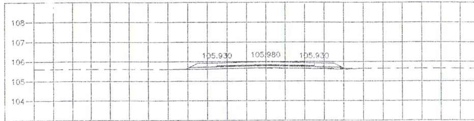
STA. 3+125.000 NGL = 105.650
