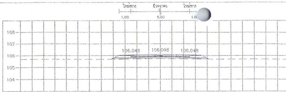
STA. 3+150.000 NGL = 105.725
