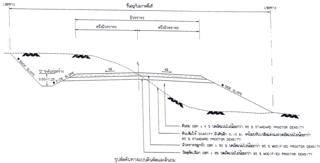
รูปตัดคันทางแบบดินคันและดินถม
