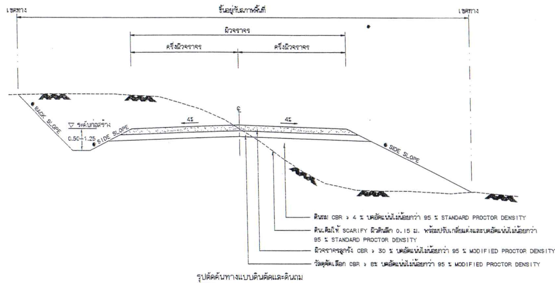
รูปตัดคันทางแบบดินเดิมและดินถม
