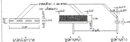
แบบขยายไม่กว้างกลางผิวพื้น คลล.
