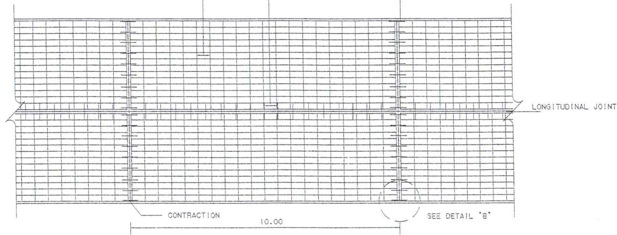
แปลนแสดงการเสริมเหล็กถนน คลล.ล.
