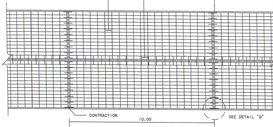
LONGITUDINAL JOINT
